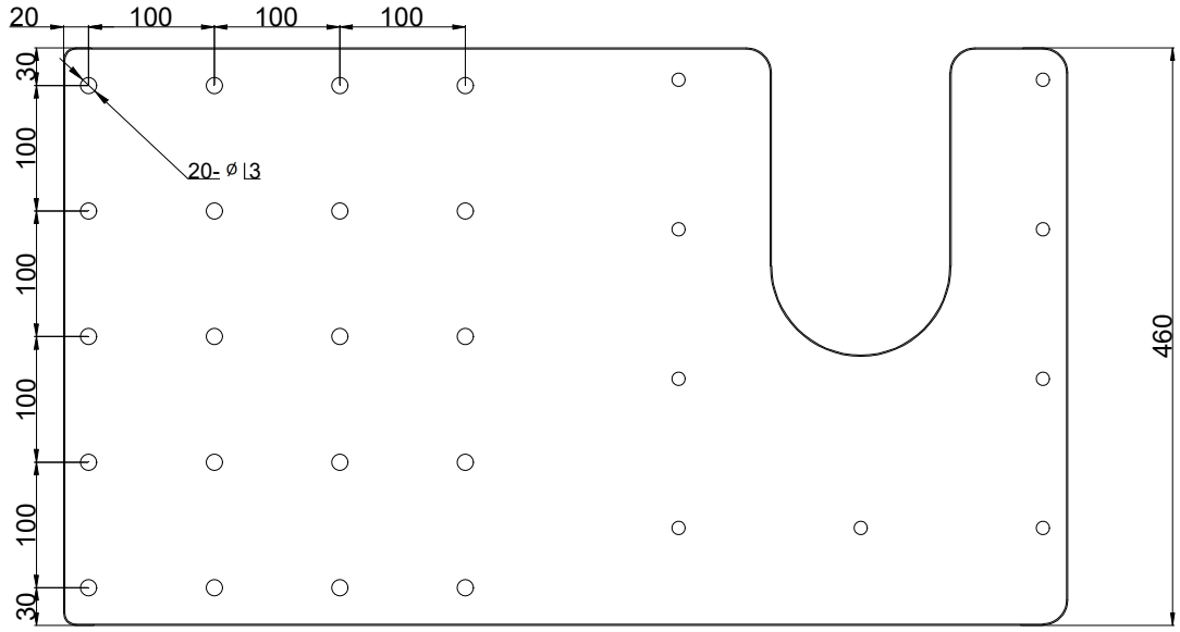
SS430 Uzatma Tabanı (800 mm)
