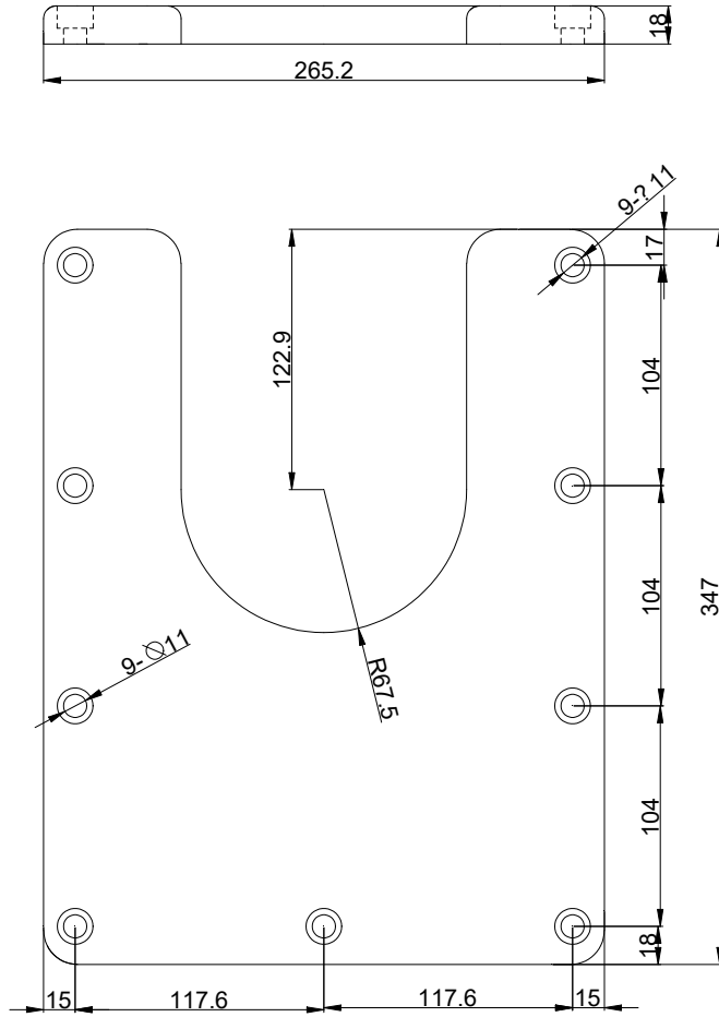
SS240 Standart Taban
