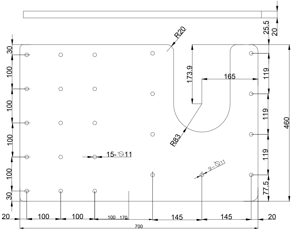
SS280 Uzatma Tabanı (700 mm)
