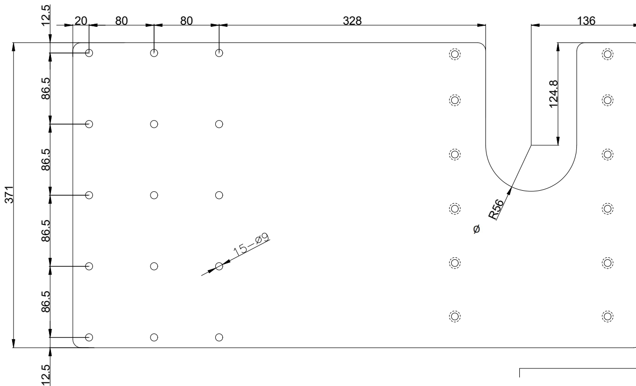
SS180 Uzatma Tabanı (700 mm)
