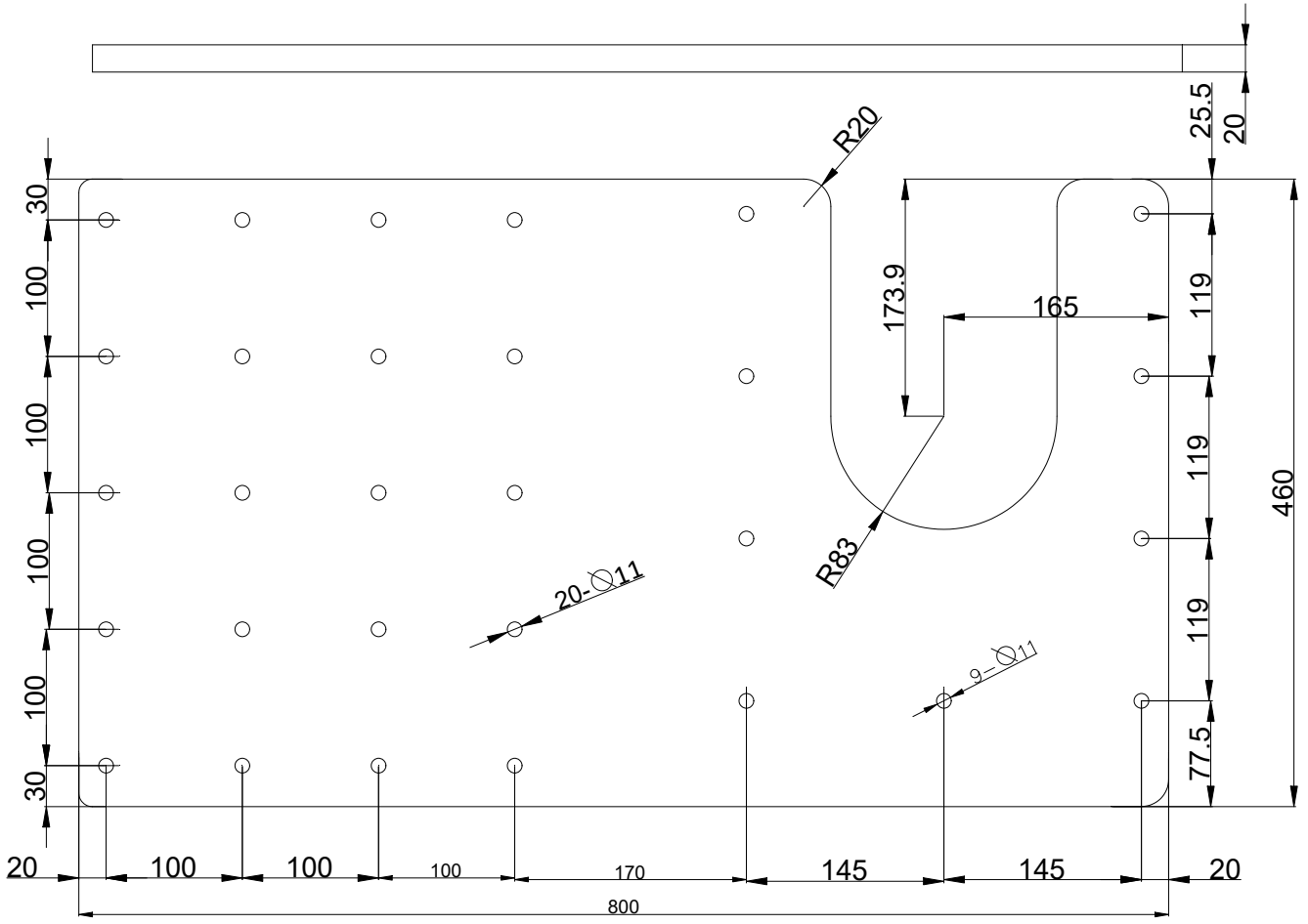
SS280 Uzatma Tabanı (800 mm)
