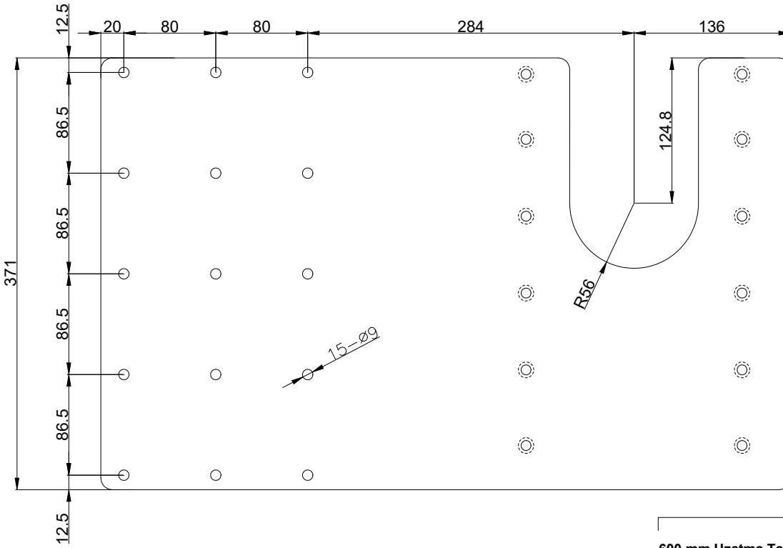
SS180 Uzatma Tabanı (600 mm)
