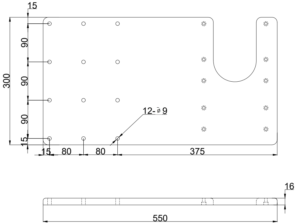
550 mm Uzatma Tabanı
