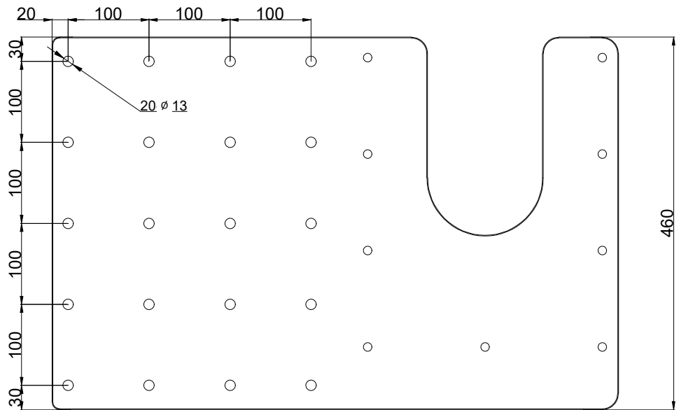
SS430 Uzatma Tabanı (700 mm)
